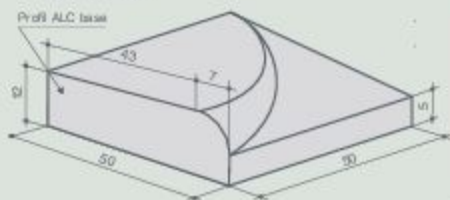
Entrée charretière profil ALC basse
