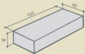
Marche bloc 40 x 100 - h = 18
